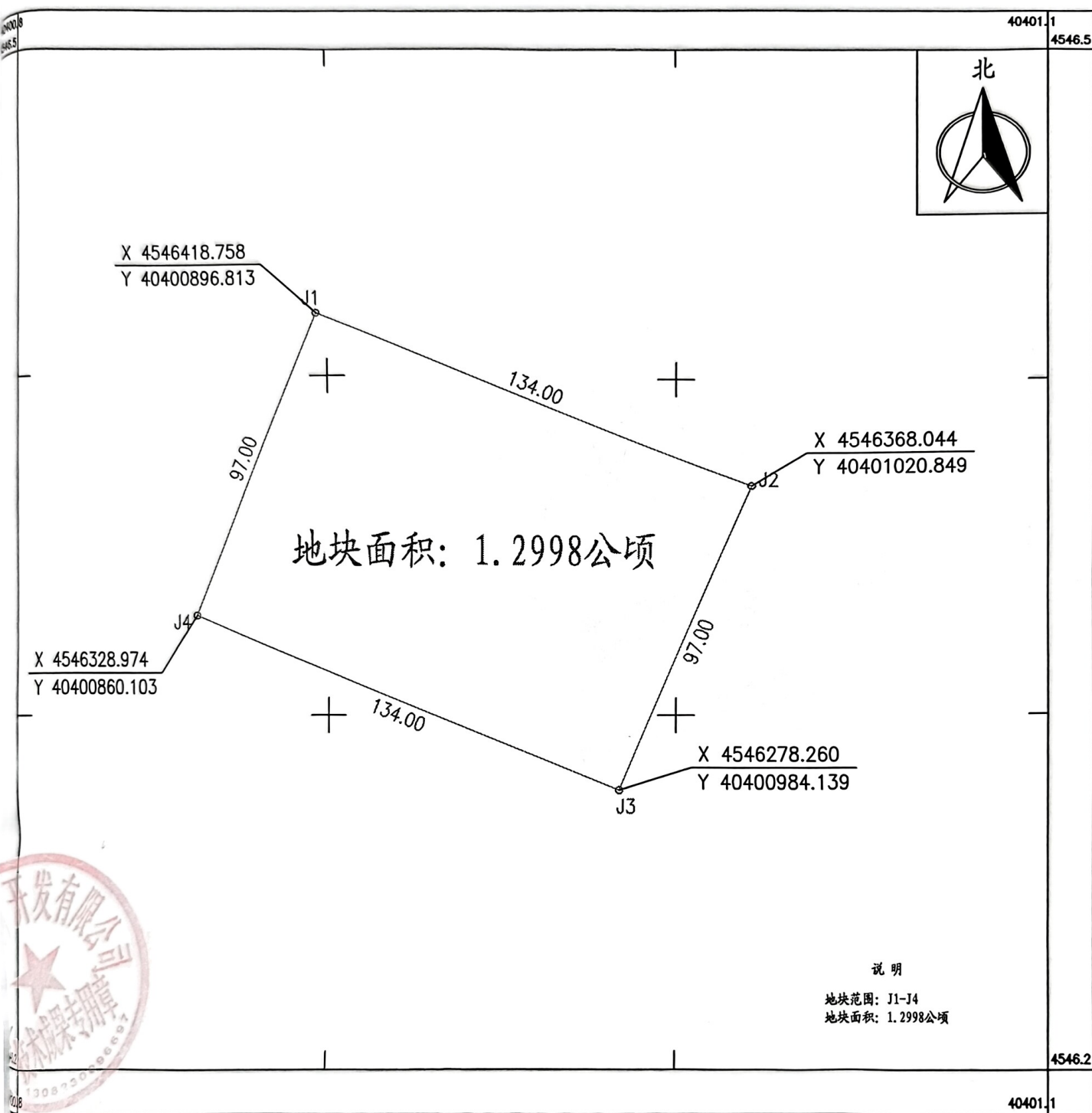
龙源平泉10万千瓦林光储氢一体化项目用地平面图
